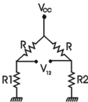
Figura 2. Puente resistivo
