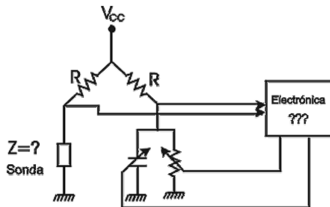
Figura 3. Puente de Impedancias adaptado al SBIB
