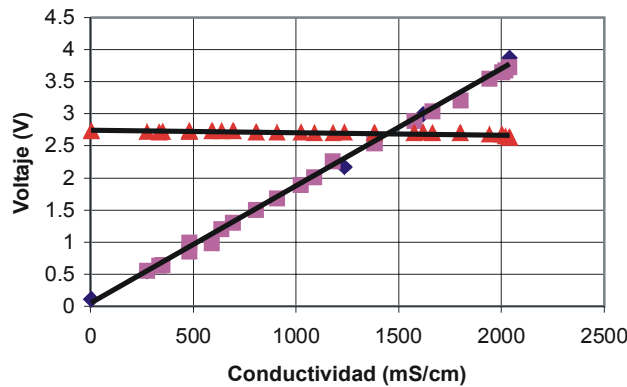
Figura 6. Independencia entre medida de humedad ( \blacktriangle ) y conductividad ( \blacklozenge ). Este experimento se realizó con distintas mezclas de líquidos orgánicos, metanol y tricloroetileno, a los que se les variaba la conductividad eléctrica añadiendo sal y manteniendo constante el valor de la cte. dieléctrica. Se puede observar que en todo el intervalo de conductividad la medida de humedad se mantiene prácticamente constante.
